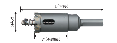
20mm~210mmまで「排出スプリング」標準装備
